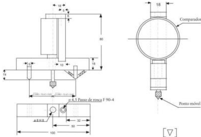
Figura 3 - Esferômetro
