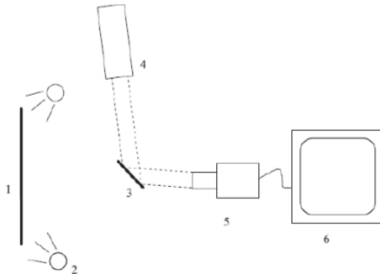
Figura 4 - Diagrama da configuração de medição de fluorescência
